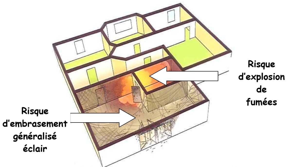
Exemple de locaux gigognes
